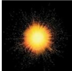
(Big Bang)
