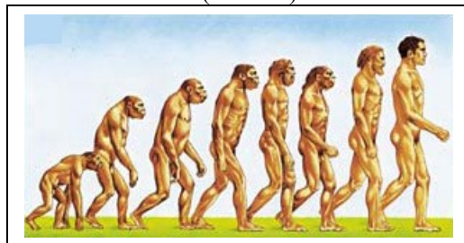
(Darwin)
